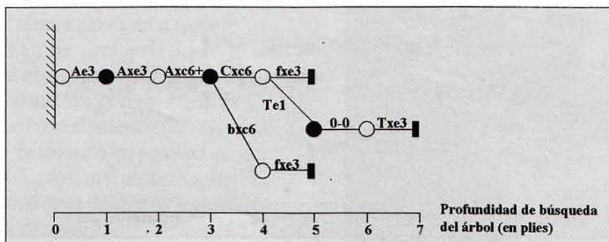
Figura 2: árbol de búsqueda para la posición del Diagrama 2.
