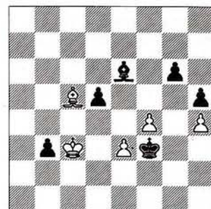
Diagrama 3: Kótov/Botvínik, 1955
