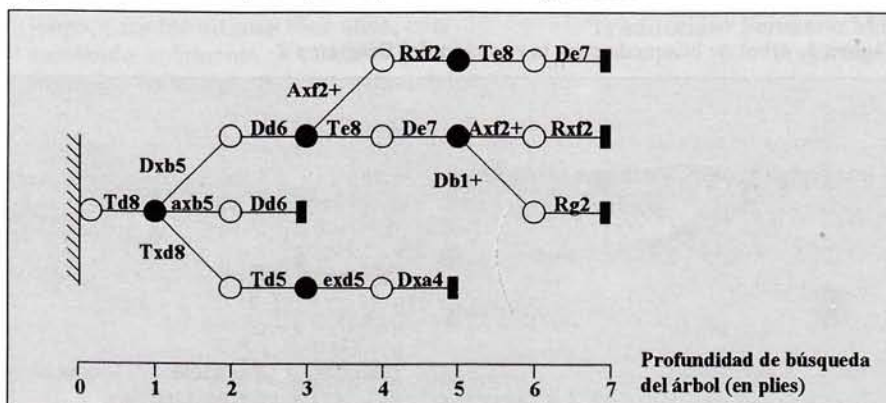
Figura 1: árbol de búsqueda para la posición del Diagrama 1.
