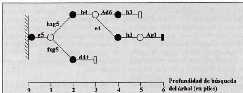
Figura 3: árbol de búsqueda para la posición del Diagrama 3.
